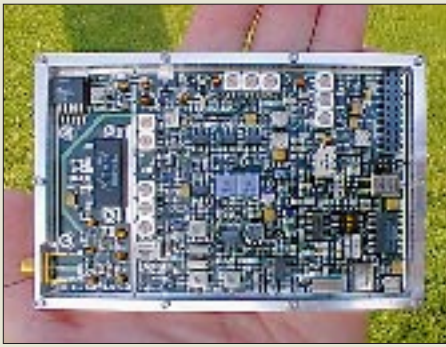
Der 70-cm-Datentransceiver RK-1A von HFB sendet mit bis zu 6 W und kann bis 19k2-FSK verarbeiten.
