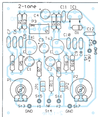
Bild 8: Bestückungsplan der Leiterplatte des Zweitongenerators
