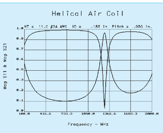
Bild 5: Eine Besonderheit von COIL besteht darin, daß Tabelle und Grafik die Ausgabedaten für Windungszahl-Zweierschritte darstellen.
