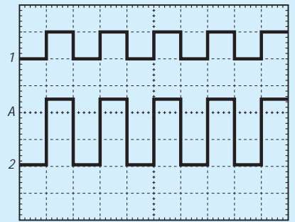
Bild 4: Dieses Oszillogramm zeigt zwei Rechteckwechselspannungen. Damit die Verschiebung der Nulllinien mit Hilfe der y-Lagesteller nicht übersehen wird, kennzeichnen digital arbeitende Oszilloskope dies im Oszillogramm durch die Ziffern 1 und 2. Diese Ziffern zeigen natürlich gleichzeitig, welche Spannung an welchem Kanal angelegt ist.
