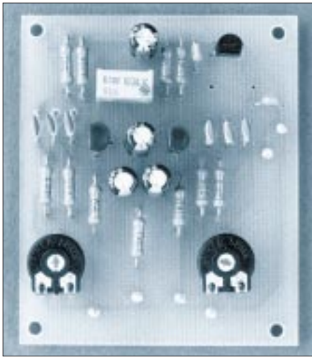
Bild 9: Eine fertige Zweitongenerator-Leiterplatte Foto: DL7UMO
