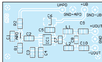
Bild 15: Für die Platine ist zweiseitiges kupferkaschirtes Material erforderlich.
