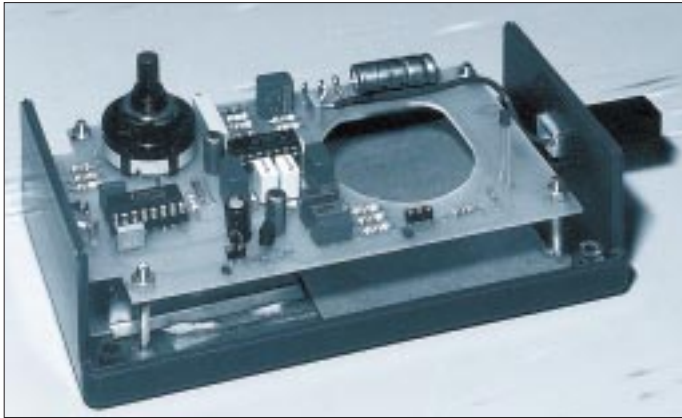
Bild 4: Die Platine wird so mit Abstandsbolzen im Gehäuse befestigt, daß darunter auch die Batterie Platz findet.
