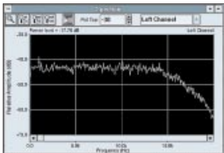
Bild 7: Frequenzgang, mit Weißem Rauschen erfaßt
