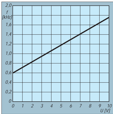
Bild 4: Wandlerkennlinie der Musterschaltung. Die Abhängigkeit U_e zu f ist linear.
