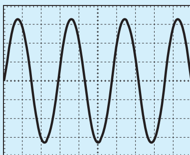
Bild 1: Durch Umschalten des Zeitmaßstabs auf einen größeren Wert bekommt man (bei gleichbleibender Frequenz der Meßspannung) mehrere Perioden der Spannung auf dem Bildschirm abgebildet.
