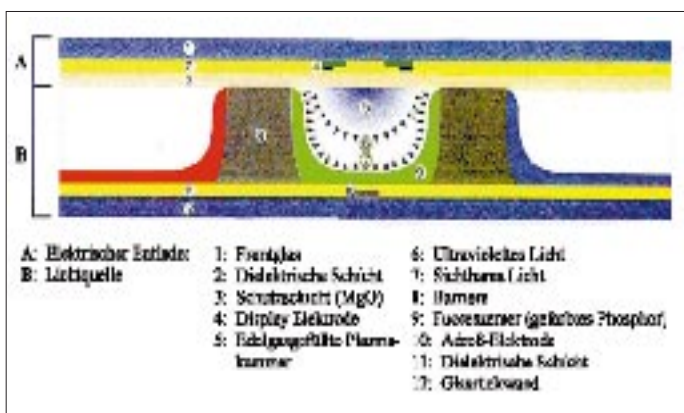
Bild 1: Das Schema zeigt den Aufbau und die Bestandteile eines PDP.
