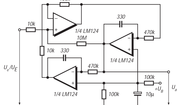
Bild 11: Aktiver 1-kHz-Bandpaß mit 40 dB Verstärkung und Q = 50
