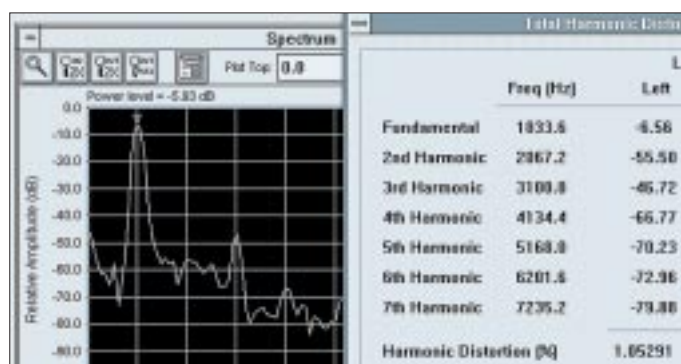
Bild 5: Klirrfaktor-Auswertung
