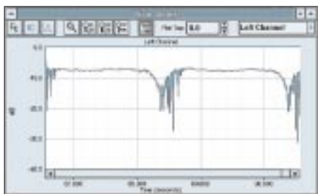
Bild 6: Frequenzgang, mit Sweep-Signal erfaßt
