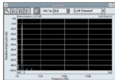
Bild 10: Empfindliche Klirrfaktormessung
