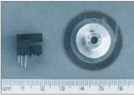
Bild 3: Der Bausatz GP1A70R mit seinen beiden Teilen. Links die Gabellichtschranke, rechts die Impulsscheibe. In der Bundbuchse ist die Imbusschraube zur Achsarretierung sichtbar.
