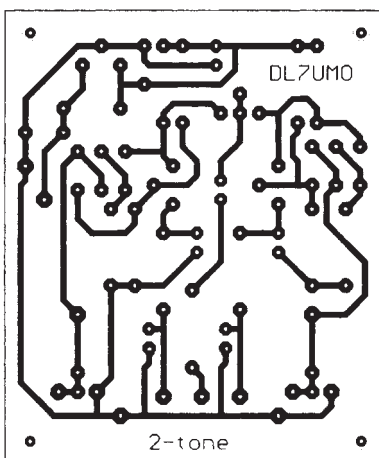
Bild 7: Leitungs- führung der Platine für den Zweiton- generator
