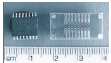
Bild 1: Wire-Wrap-Sockel DIL16. Oben die dünnen, unten die dicken Stifte. Bild 2: Der Adapter SO16schmal>DIP16 in Schräglage Bild 3: Blick auf die Oberseite des Adapters, daneben ein TSA6060.
