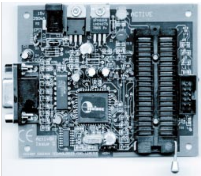
Bild 4: Das Programmiergerät
