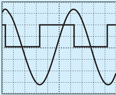
Bild 3: Ein Zweikanal-Oszilloskop erlaubt wahlweise eine oder zwei Spannungen gleicher Frequenz gleichzeitig auf dem Bildschirm darzustellen. Hier zeigt das Oszillogramm eine sinusförmige Wechselspannung und eine Rechteckspannung mit positiven Impulsen.
