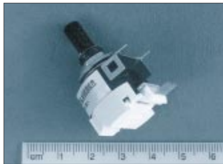
Bild 4: Inkrementaler Geber M101B-100. Die Rückplatte trägt neben den vier stabilen Kontaktstiften auch die interne Elektronik.
