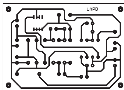
Bild 18: Das Platinenlayout für die Spannungserzeugung mit dem MAX1771
