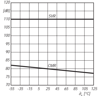
Bild 8: Betriebsspannungs- und Gleichtaktunterdrückung über der Einsatztemperatur
