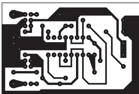
Bild 2: Platinenlayout
