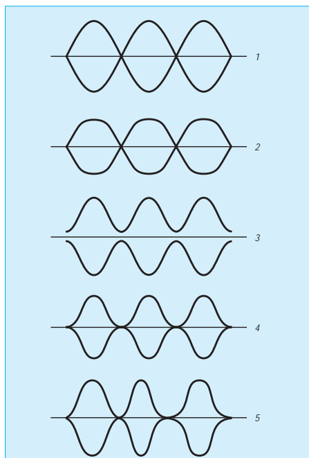
Bild 1: Bei korrekter Linearität kreuzen sich beim Zweitontest die Sinushalbwellen der Hüllkurve scharf auf der x-Achse
