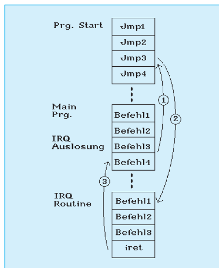
Bild 1: IRQ-Ablauf
