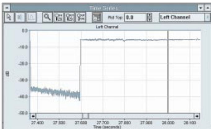
Bild 8: Ermittlung des Störabstands (Differenz zwischen Talsohle und Dachwert)
