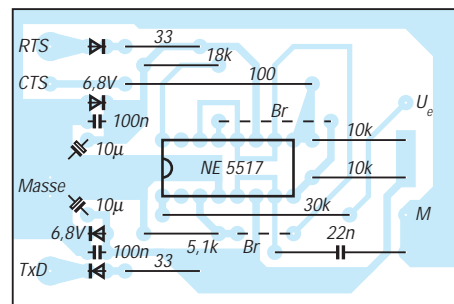
Bild 3: Bestückungsplan
